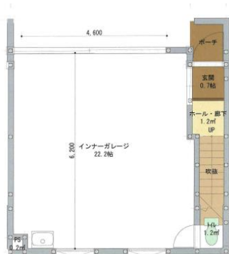
1階平面図
