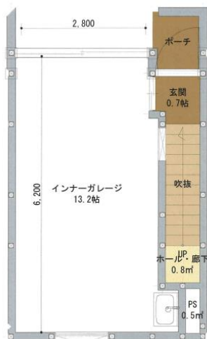
1階平面図
