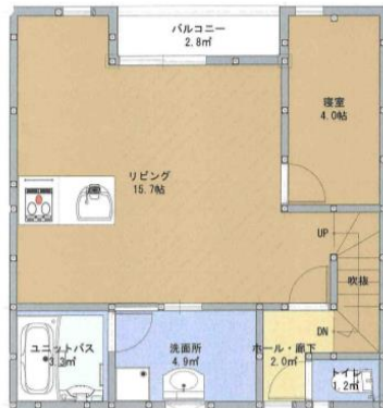
2階平面図
