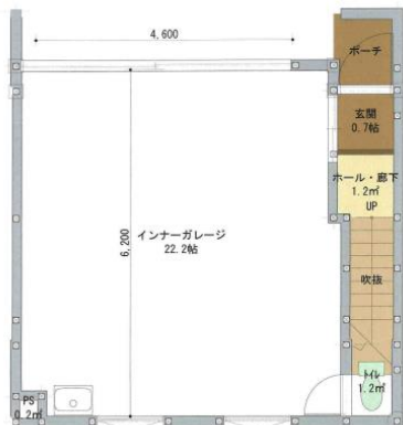
1階平面図
